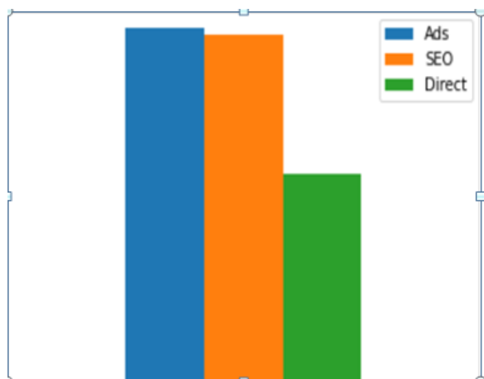
Figure. 3 Browser
