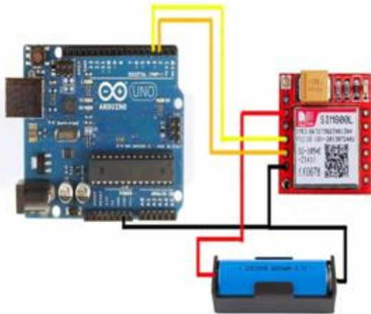
Figure 20. GSM module
